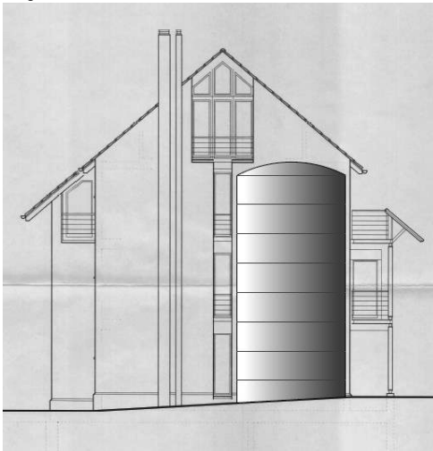
Ansicht West
