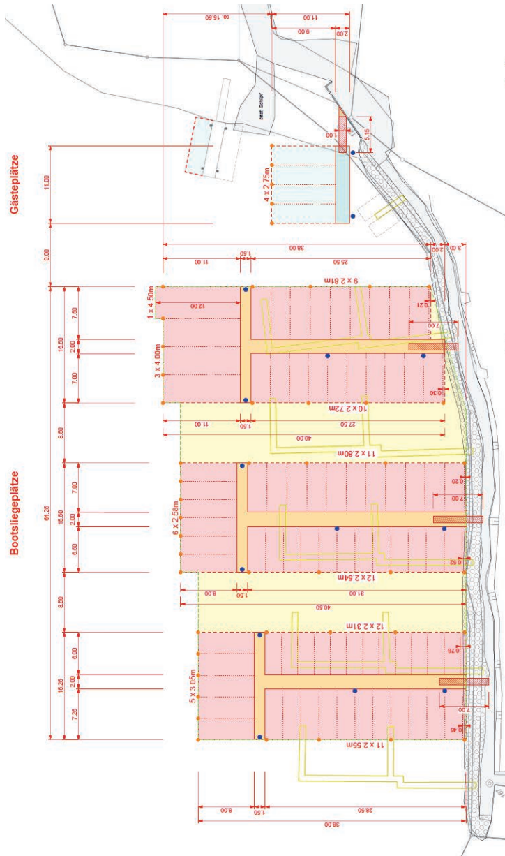
Abbildung 1: Grundriss Bootssteganlage
