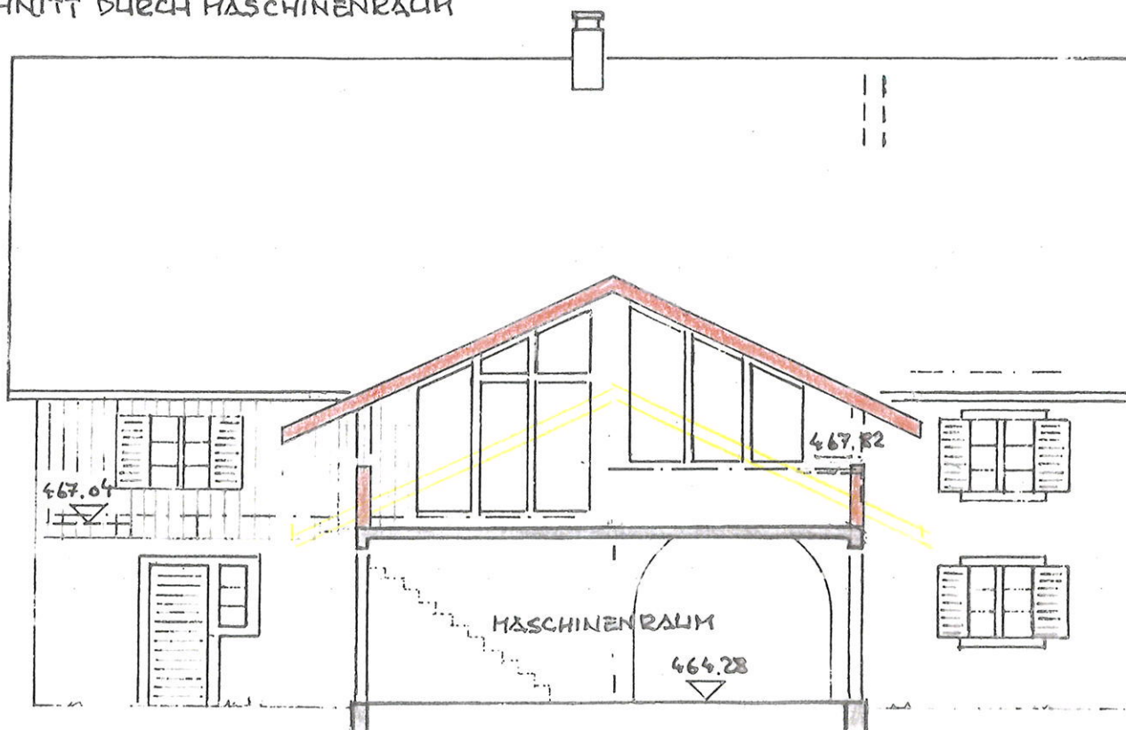
SCHNITT DURCH MASCHINENRAUM
